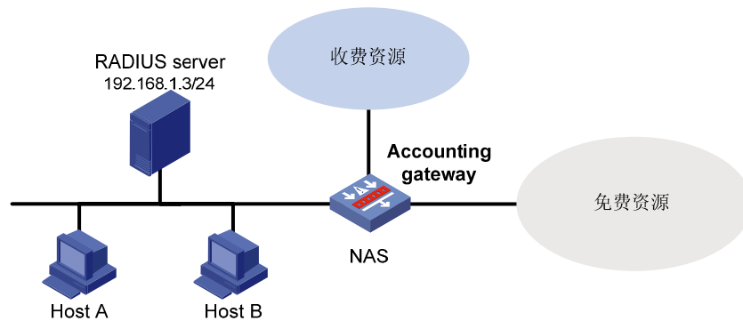
图1-2 用户流量计费典型配置组网图
