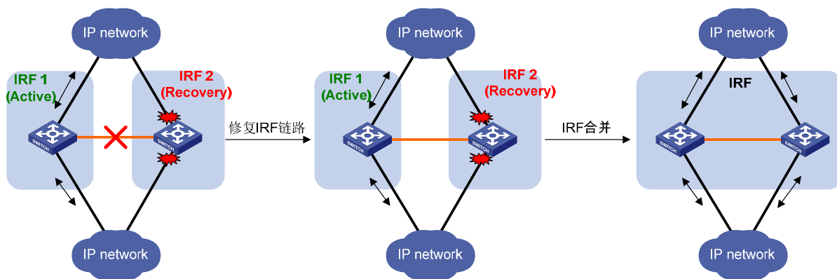
图1-10 MAD 故障恢复（IRF 链路故障）
