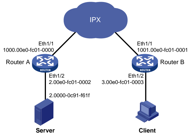
图1-1 IPX 配置组网图
