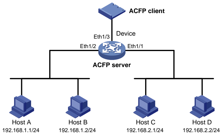
图1-2 ACFP 典型配置组网图
