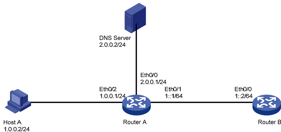
图1 IPv6 NAT-PT 与 DNS-ALG 配合功能的配置组网图
