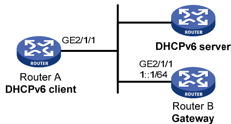
图4-3 DHCPv6 无状态配置组网图
