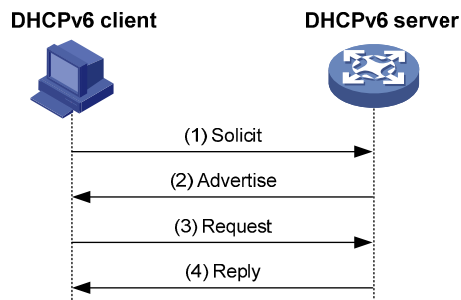
图1-2 交互四个消息的分配过程
