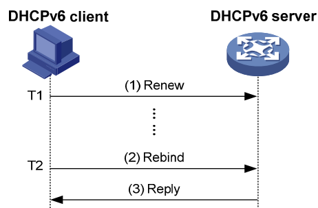
图1-4 通过 Rebind 更新地址/前缀租约
