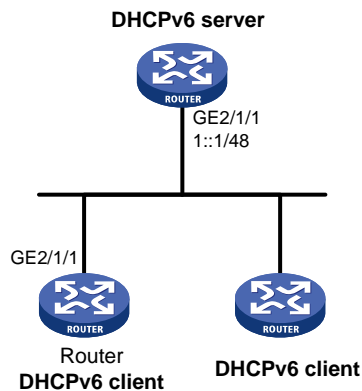
图4-1 DHCPv6 客户端申请地址及网络参数配置组网图
