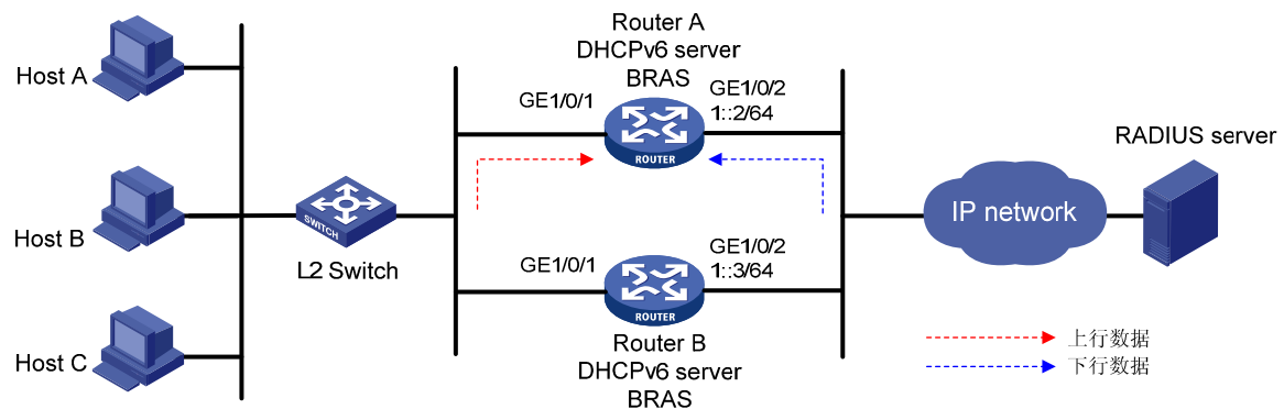
图2-4 DHCPv6 服务器辅助路由组网图
