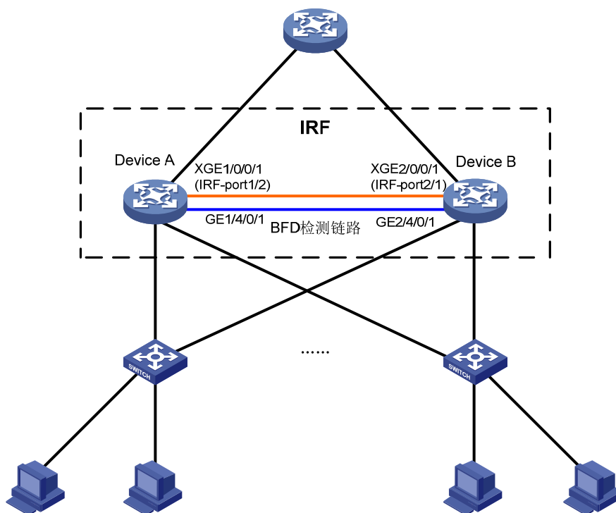
图1-13 在 SR8800-F 上组建 IRF 典型配置组网图（BFD MAD 检测方式）
