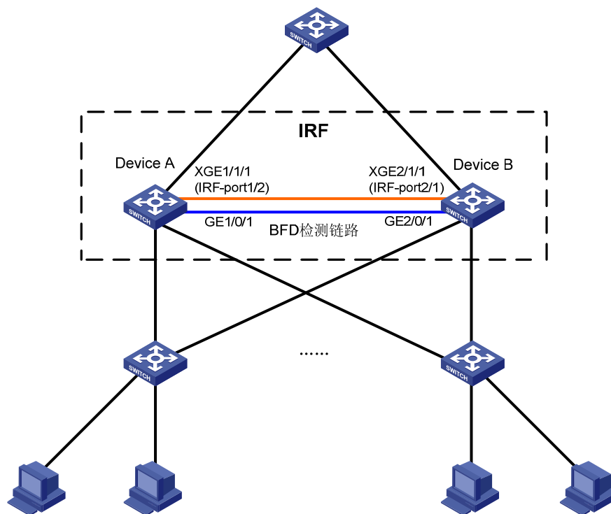
图1-14 IRF 典型配置组网图（BFD MAD 检测方式）
