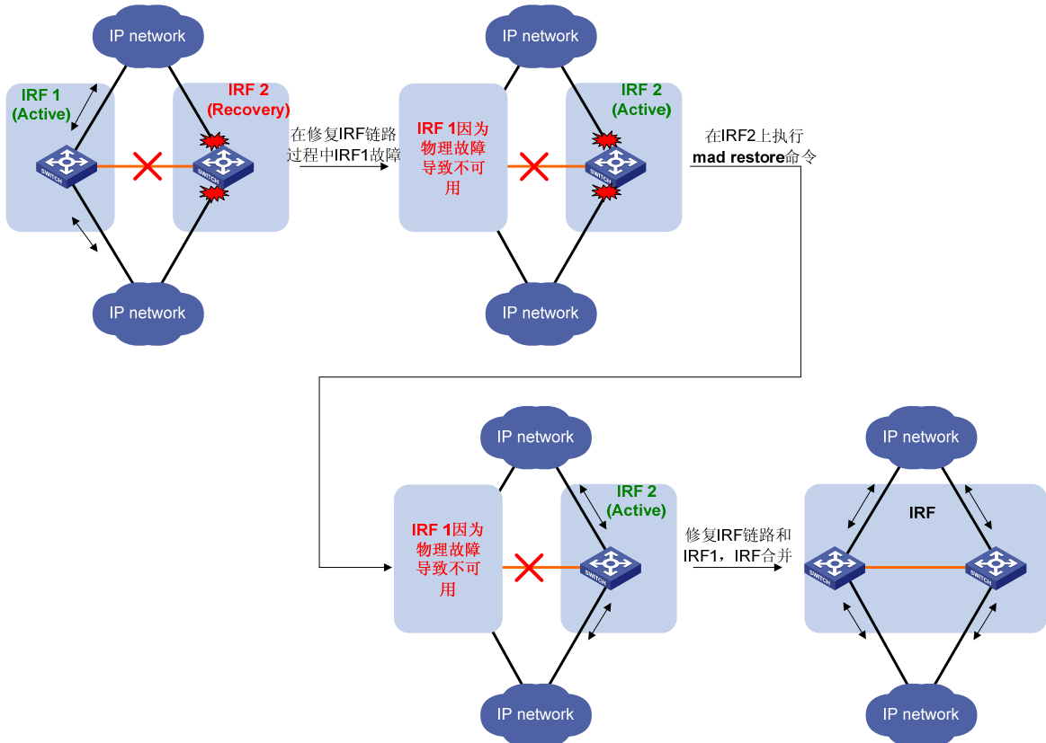
图1-12 MAD 故障恢复（IRF 链路故障+Active 状态的 IRF 故障）
