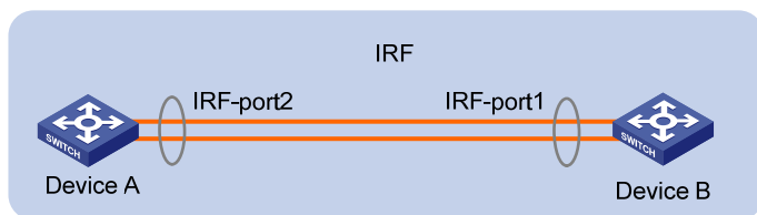
图1-4 IRF 物理连接示意图
