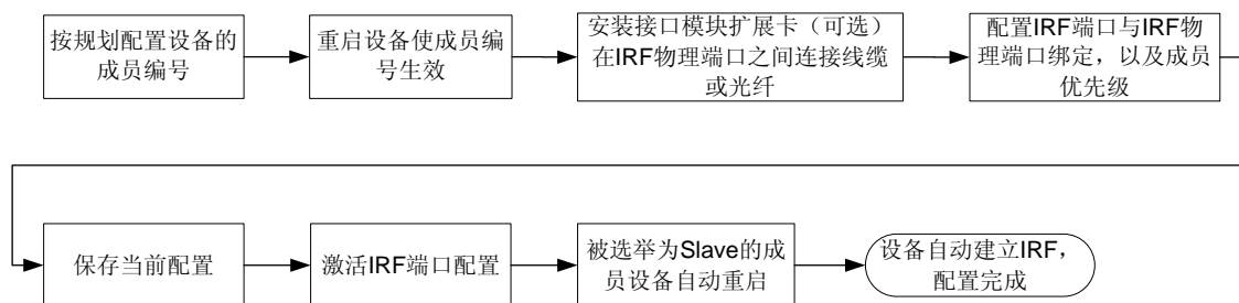
图1-6 IRF 配置流程图
