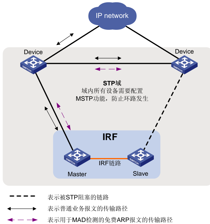
图1-10 ARP MAD 检测组网示意图
