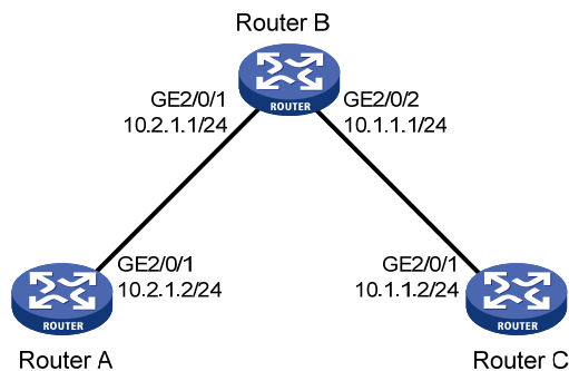
图1-16 NQA 联动配置组网图
