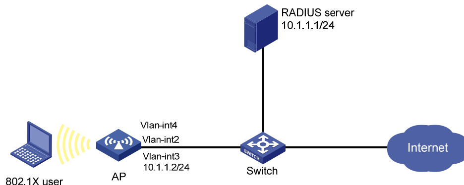
图1-19 802.1X 用户 RADIUS 认证、授权和计费配置组网图
