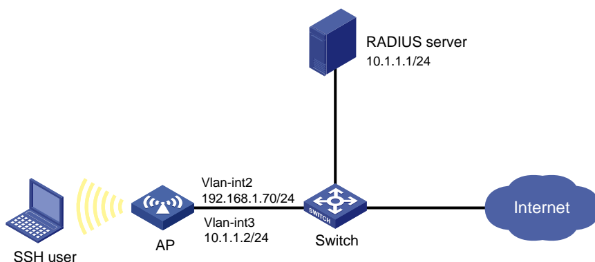
图1-11 SSH 用户 RADIUS 认证/授权配置组网图
