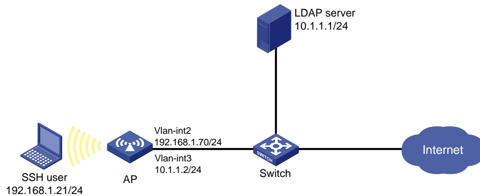
图1-14 SSH用户LDAP认证配置组网图
