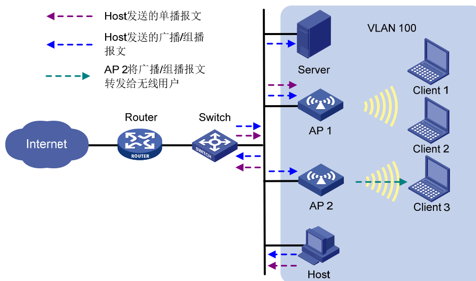
图1-3 有线用户报文路径转发示意图
