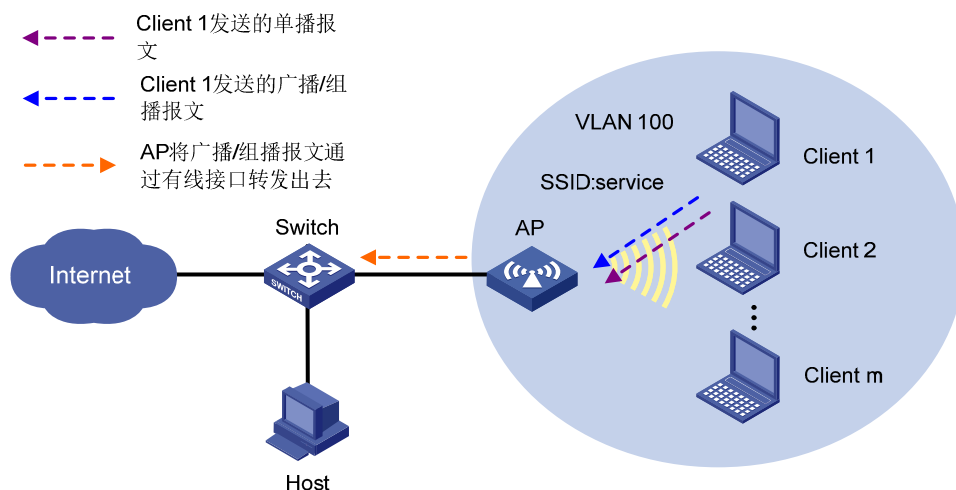
图1-1 报文路径转发示意图
