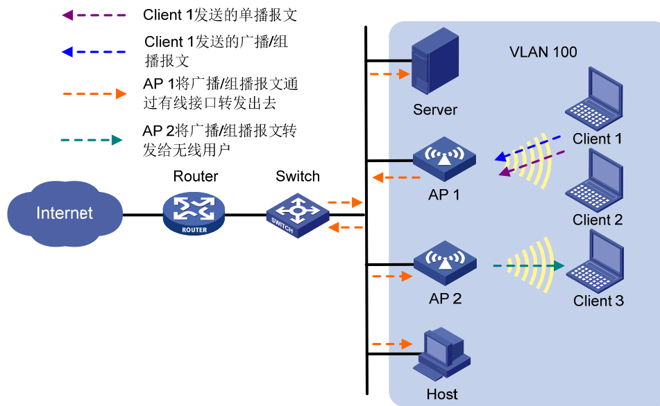
图1-2 无线用户报文路径转发示意图
