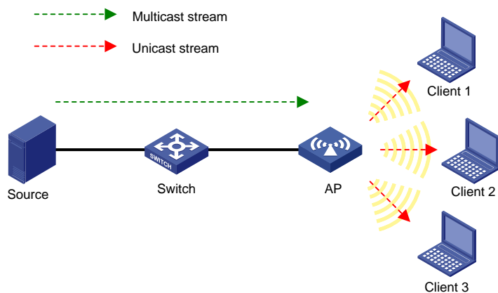
图1-1 开启组播优化后数据传输示意图
