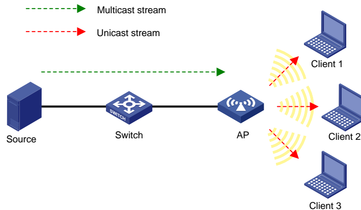
图1-2 组播优化基本组网图
