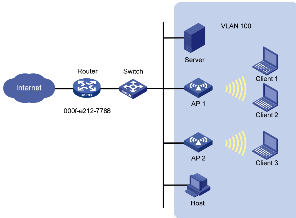
图1-5 基于 VLAN 的用户隔离配置组网图
