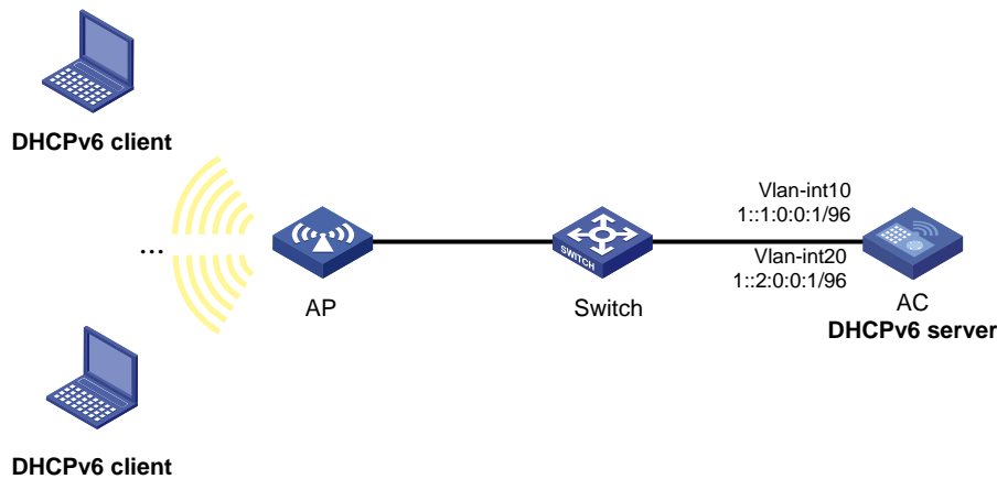
图2-6 DHCPv6 动态分配 IPv6 地址组网图
