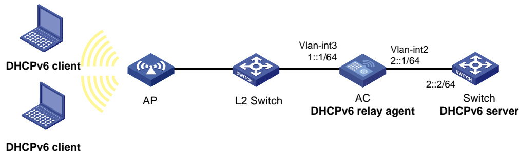
图3-3 DHCPv6 中继组网图
