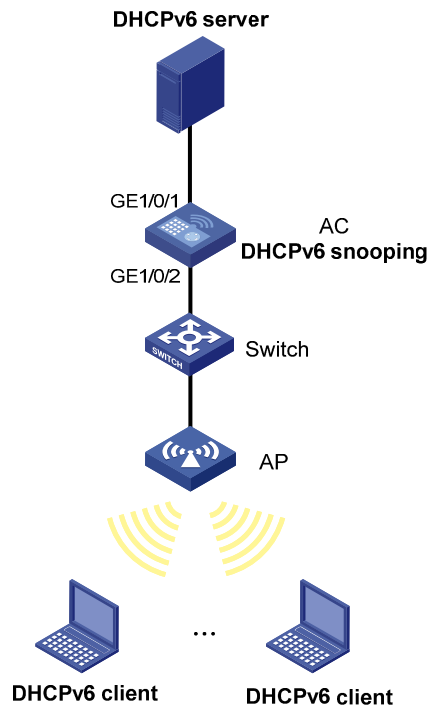
图5-4 DHCPv6 Snooping 组网示意图
