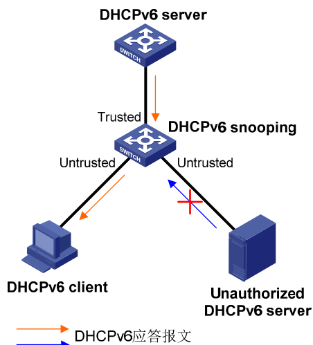
图5-1 信任端口和非信任端口
