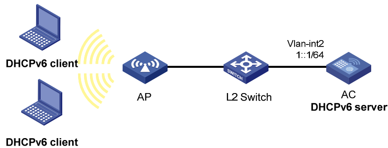
图2-5 DHCPv6 服务器配置组网图
