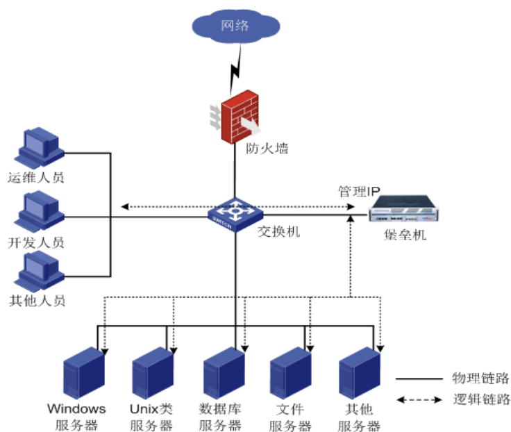
图2-1 运维审计系统网络图
