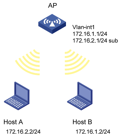
图1-5 IP 地址配置组网图
