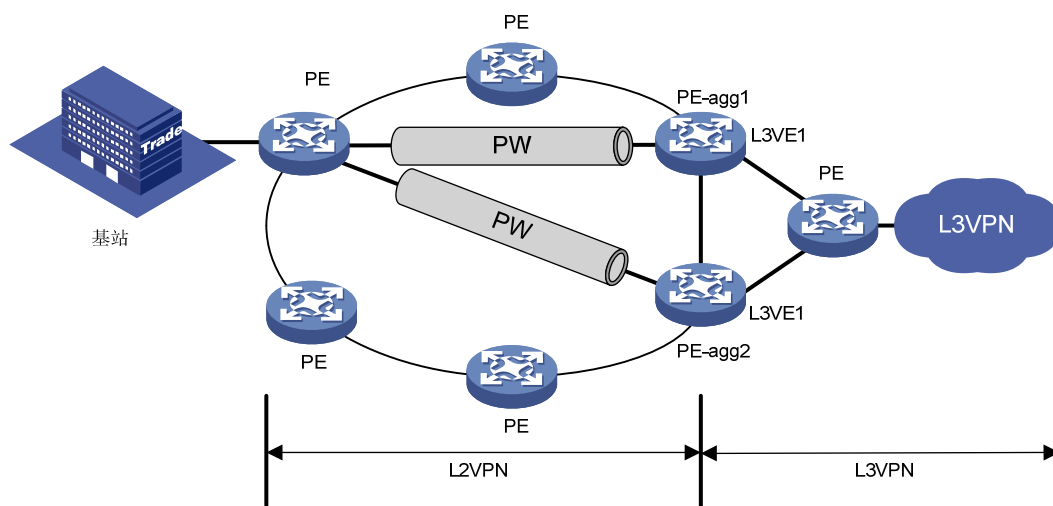
图2-6 ND 直连路由通告组网图
