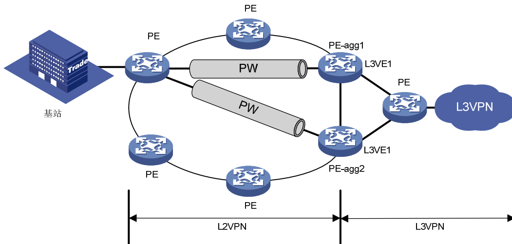
图2-5 ND 泛洪抑制组网图
