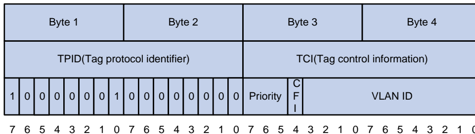
图8-3 802.1Q 标签头
