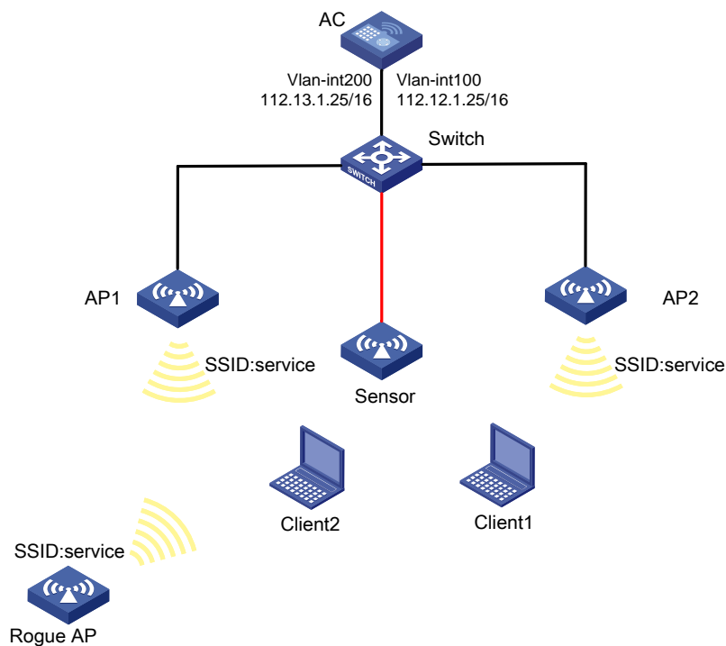
图1 WIPS 组网图
