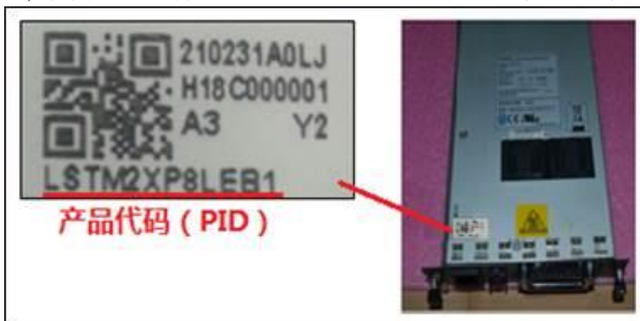
图 18 电源模块序列号标签示意图
