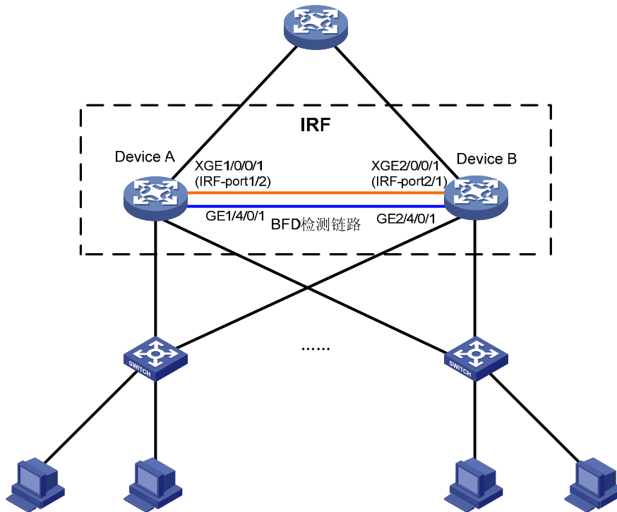
图1-13 在 SR8803-X-S、SR8806-X-S 或 SR8810-X-SSR8800-F 上组建 IRF 典型配置组网图(BFD MAD 检测方式)
