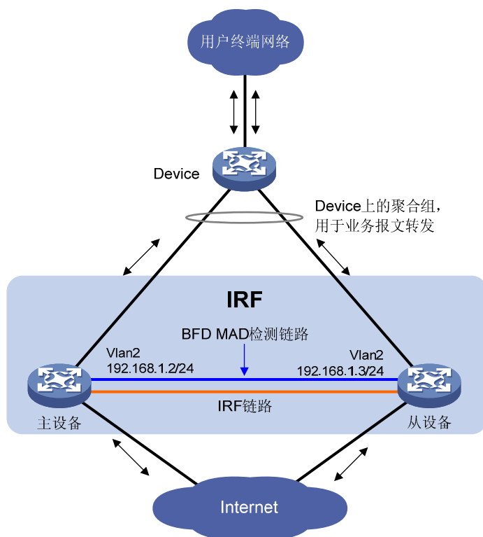
图1-9 BFD MAD 检测组网示意图
