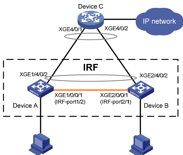
图1-12 在 SR8800-F 上组建 IRF 典型配置组网图（LACP MAD 检测方式）
