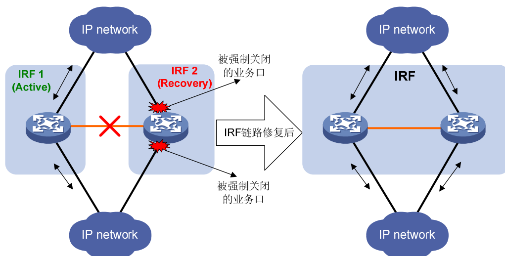
图1-10 MAD 故障恢复（IRF 链路故障）
