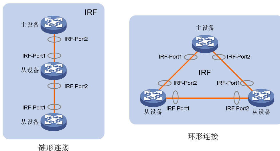
图1-7 IRF 连接拓扑示意图
