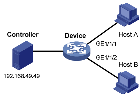
图1-8 接口类型 OpenFlow 配置组网图
