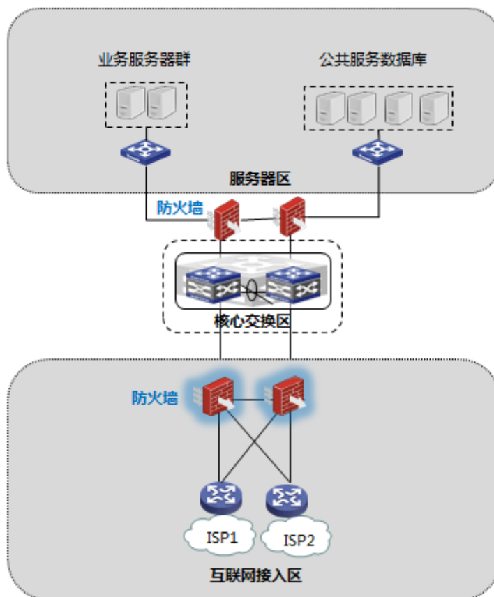
H3C SecPath F100/F1000 IT 专用防火墙组网应用示意图
