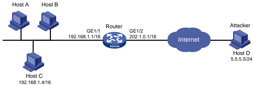
图1-2 黑名单配置典型组网图
