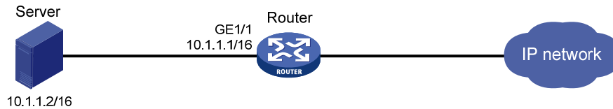
图1-3 流量统计配置典型组网图
