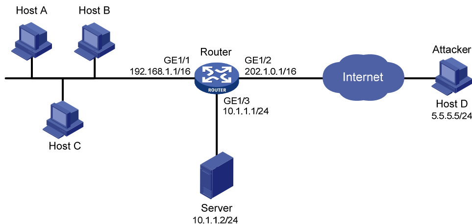
图1-1 接口上的攻击防范配置典型组网图
