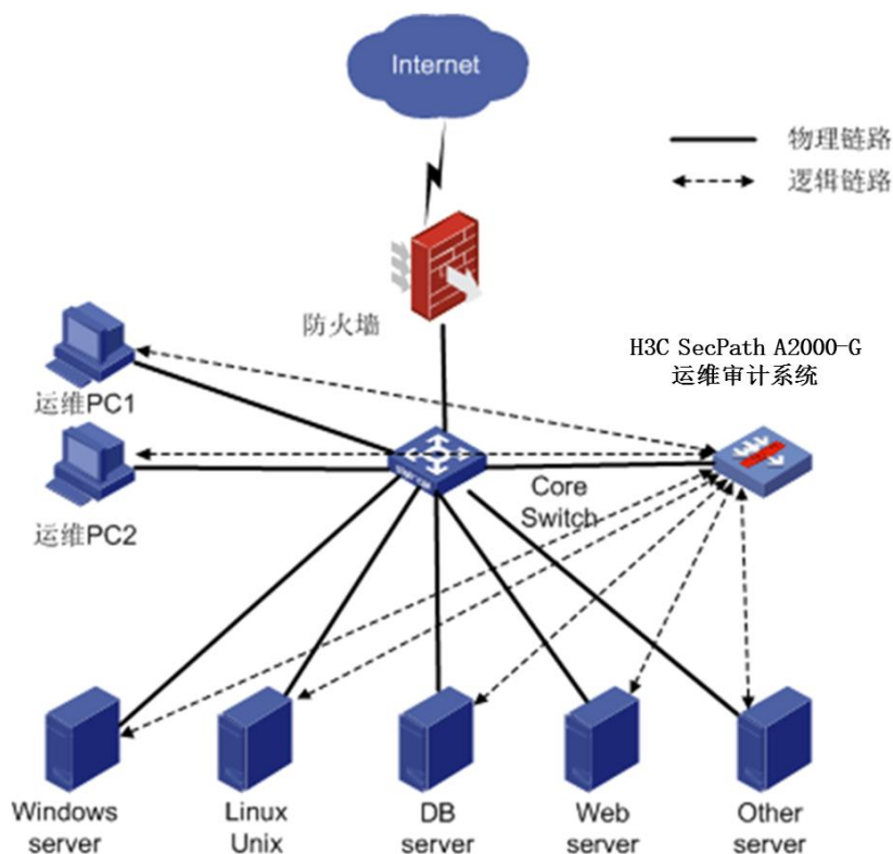
H3C SecPath A2000-G 运维审计系统应用组网图
