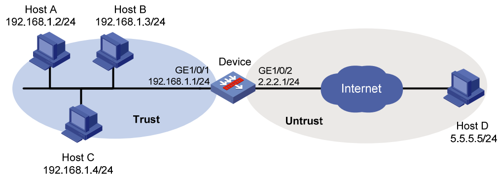
图1-2 单通道模式带宽管理典型配置组网图
