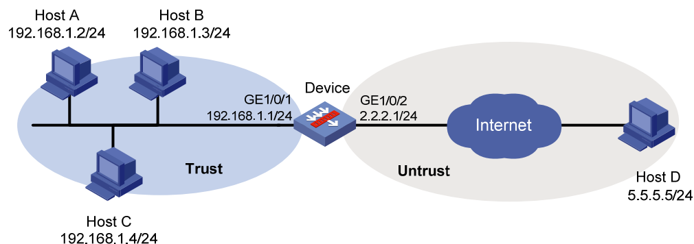
图1-3 父子通道模式带宽管理典型配置组网图
