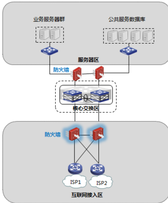
H3C SecPath F100-C-A5 组网应用示意图
