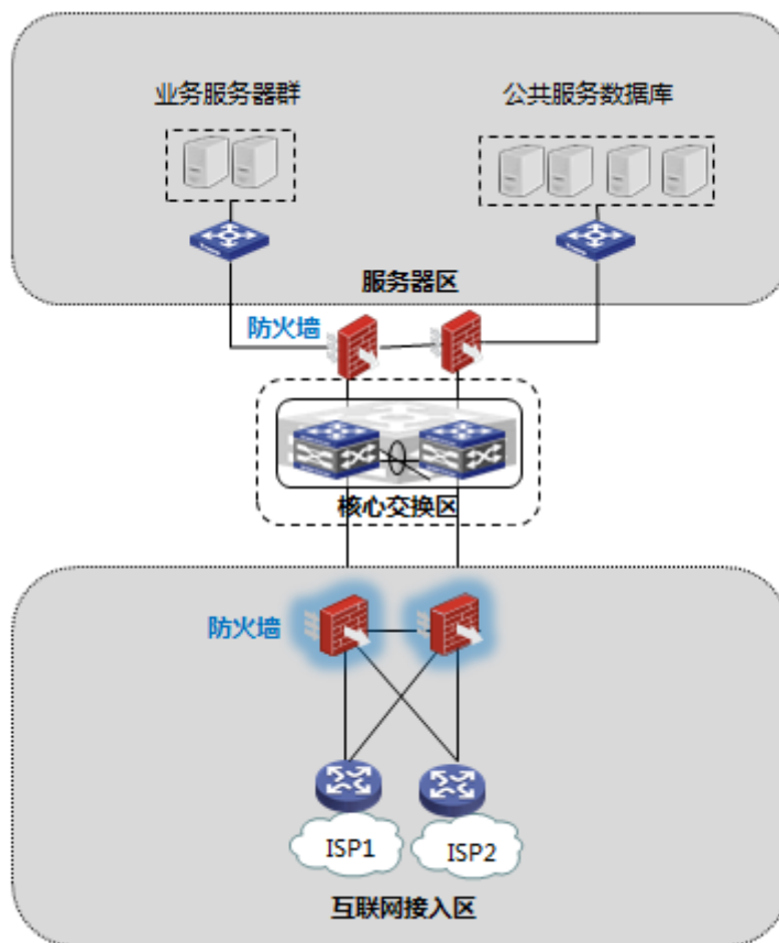
H3C SecPath F100-C-A3 组网应用示意图
