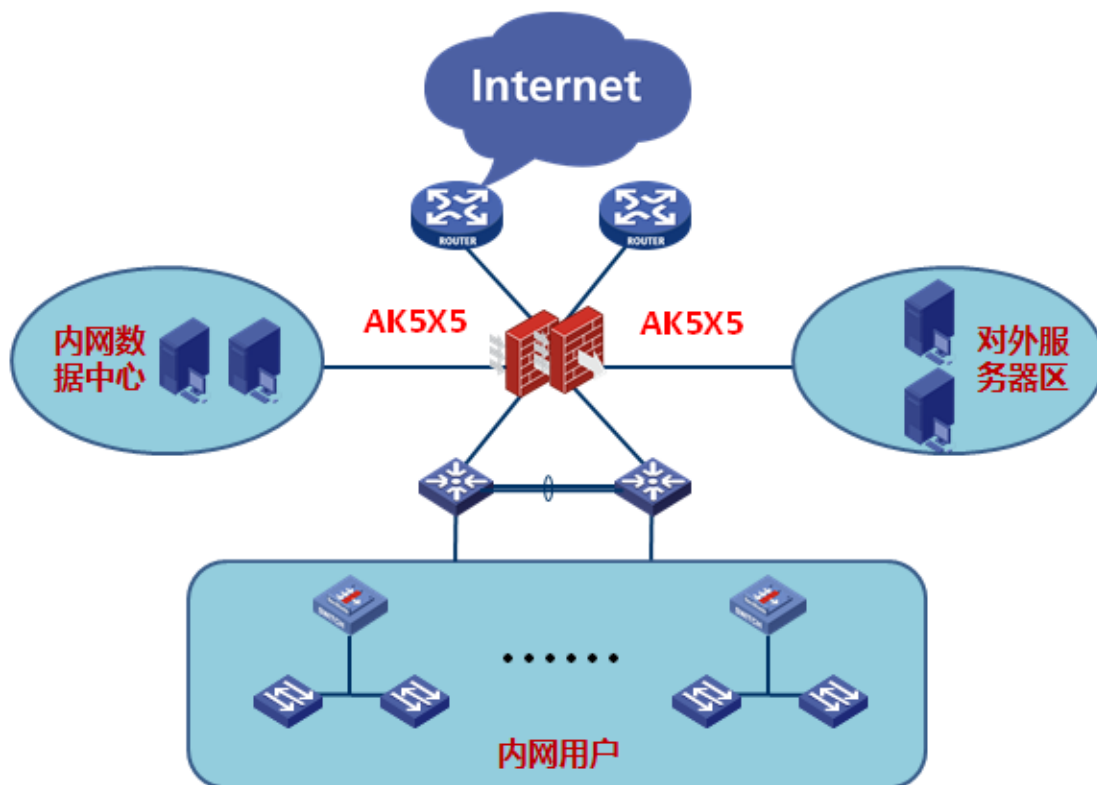
H3C SecPath F5000-AK515 组网应用示意图
