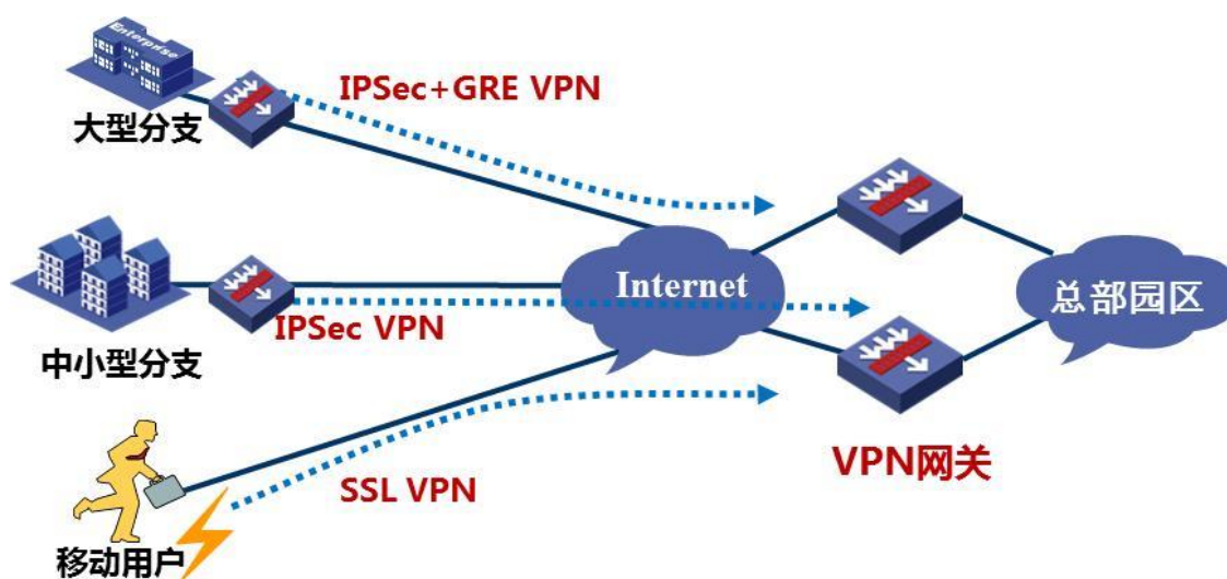
图1-12 VPN 应用组网图
