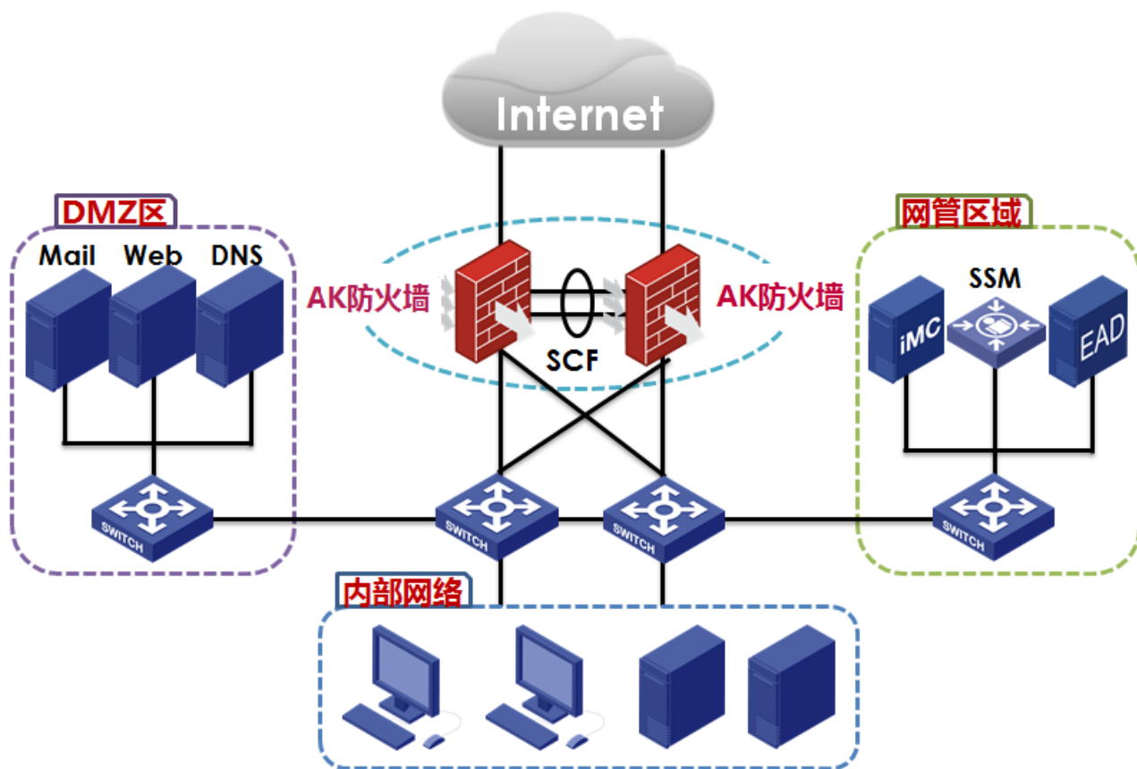
H3C SecPath F1000-AK12X2/AK13X2 系列组网应用示意图
