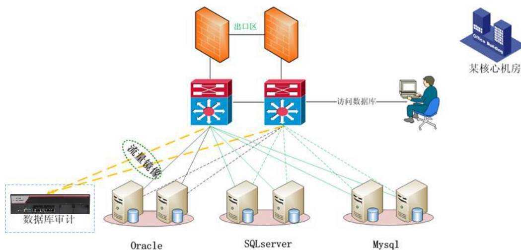
H3C SecPath D2000-AK 系列数据库审计系统部署图
