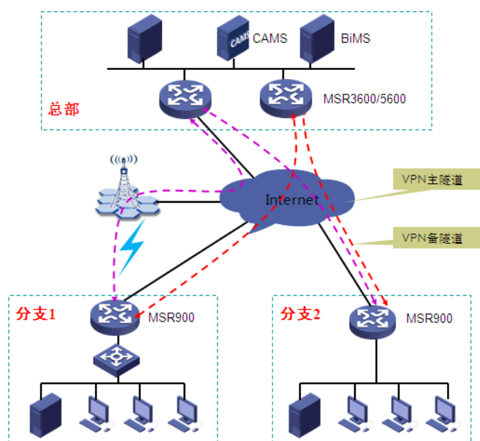
商业连锁企业 VPN 应用示意图
