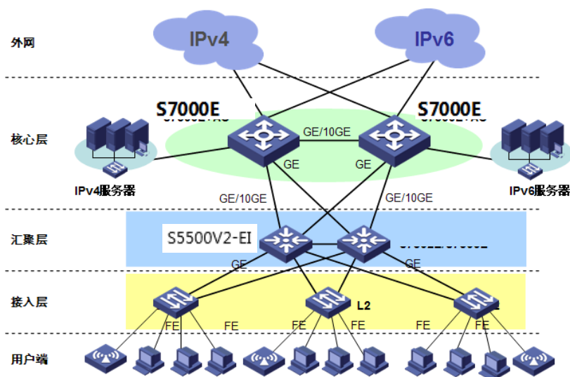
图 3 H3C S7000E 在园区网的应用
