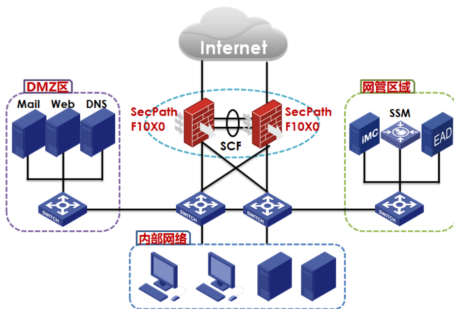
H3C SecPath F10X0 系列组网应用示意图
